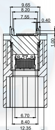
剖面 B-B 缩放 1:1
