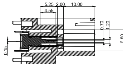
剖面 A-A 缩放 1:1
