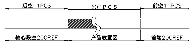
包装示意图:
