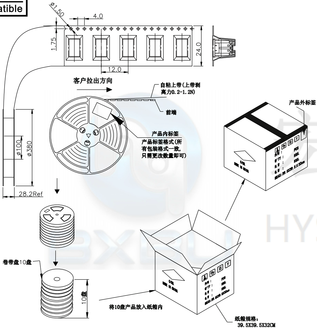
包装示意图:
