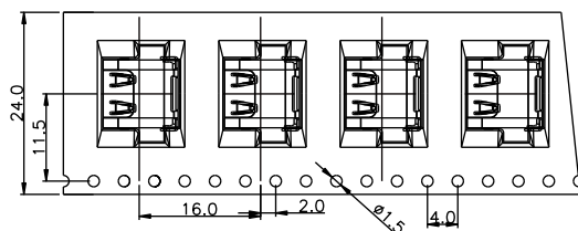
① 产品入载带示意图
