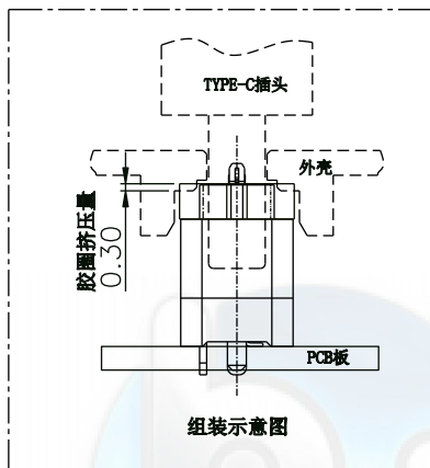
组装示意图
