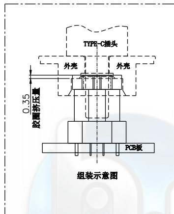
组装示意图
