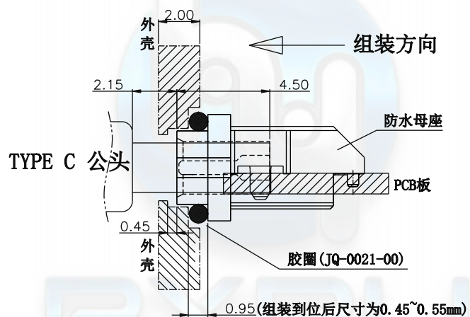
组装示意图(胶圈未挤压状态)
