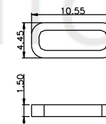
防水圈图示
