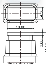
装前塞示意图
