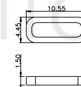
防水圈图示
