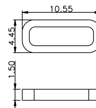
防水圈图示
