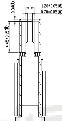
剖视图
