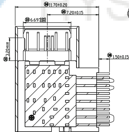
剖视图
