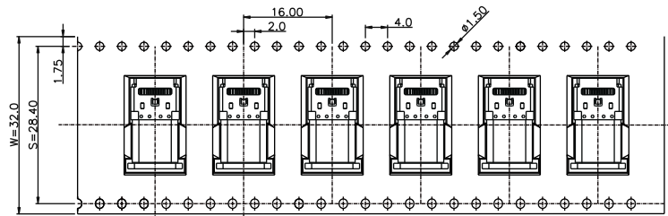
① 产品入载带示意图
