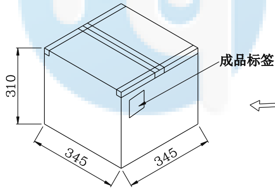
⑤ 外箱封箱示意图
