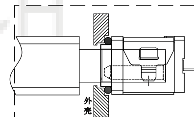
组装示意图
