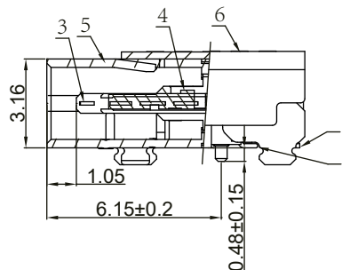
SECTION A-A(剖视图A-A) SCALE 2:1 (比例 2:1)
