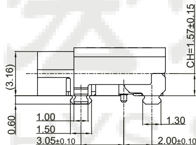
SECTION A-A(剖视图A-A) SCALE 2:1 (比例 2:1)
