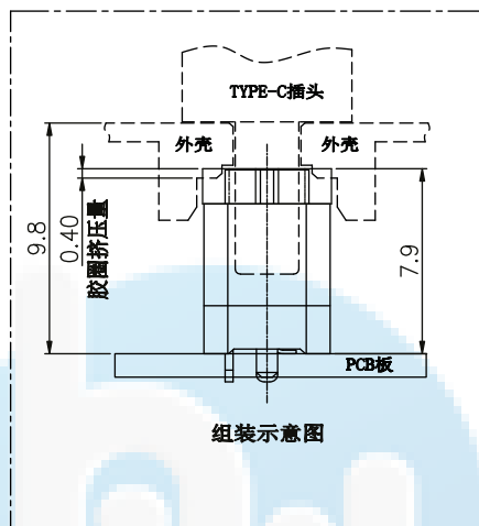
组装示意图
