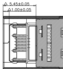
截面B-B
