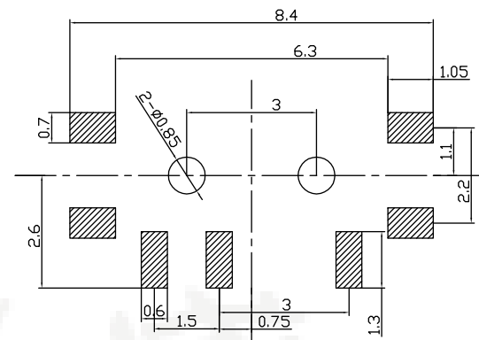
安装参考图
