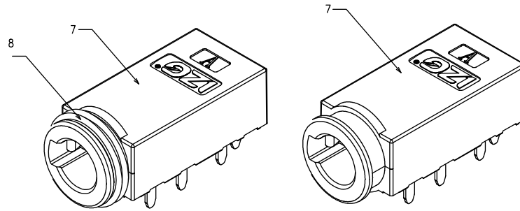
带防水圈 3D VIEW 不带防水圈
