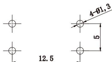
PCB. 焊接图
