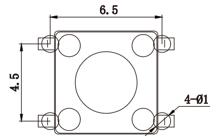
PCB板安装尺寸
