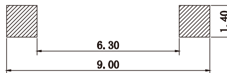
PCB. 焊接图
