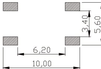
PCB. 焊接图
