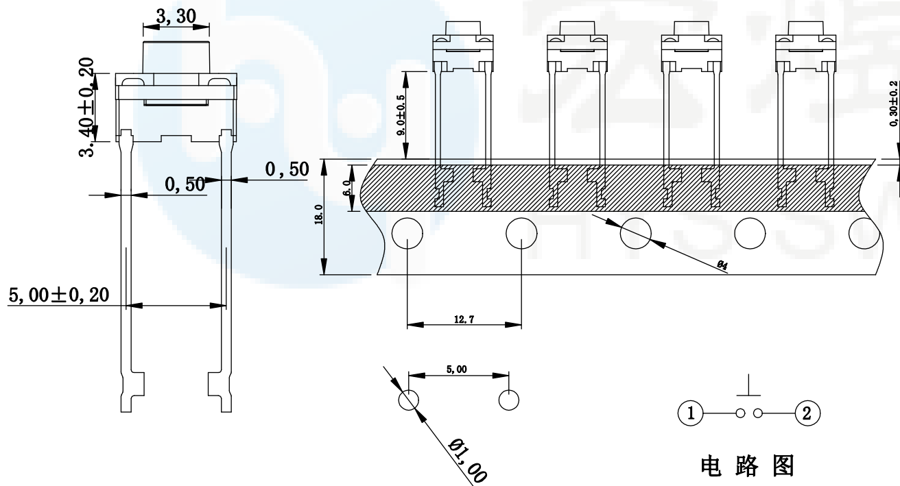
PCB. 焊接图
